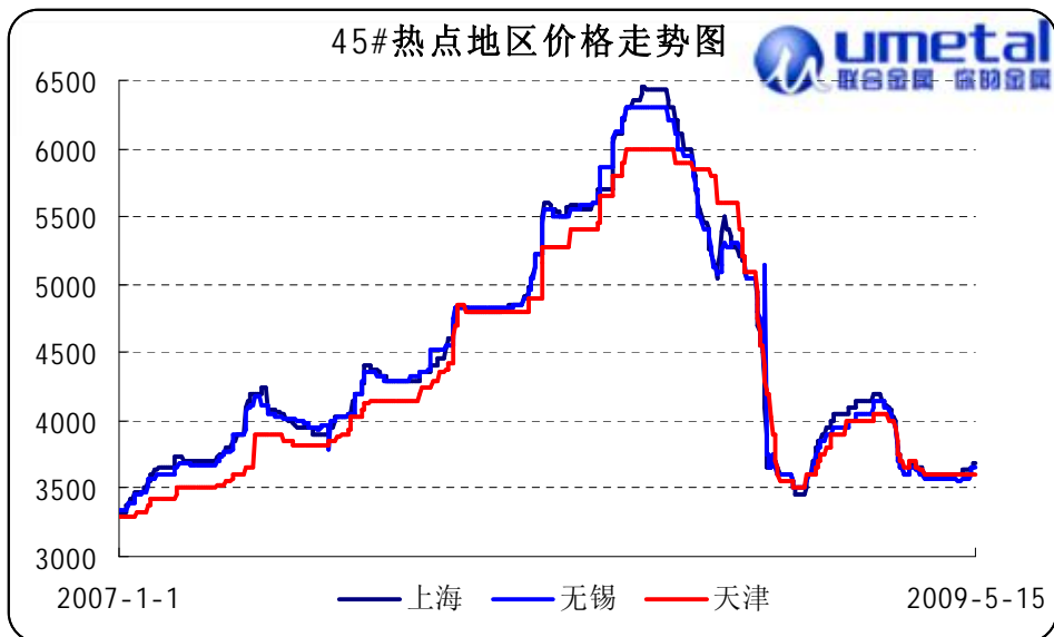
合结钢产品价格走势图
