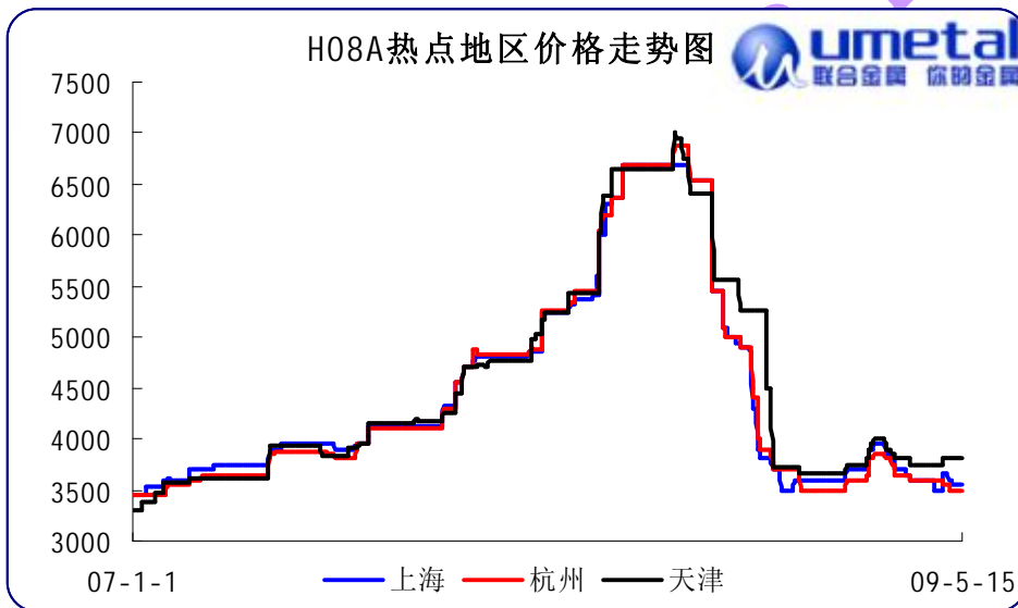
焊线产品价格走势图
